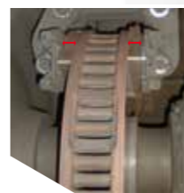
Vérification de l'usure des freins / Brake wear check
