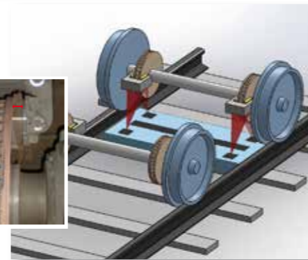
Vérification de l'usure des freins / Brake wear check
