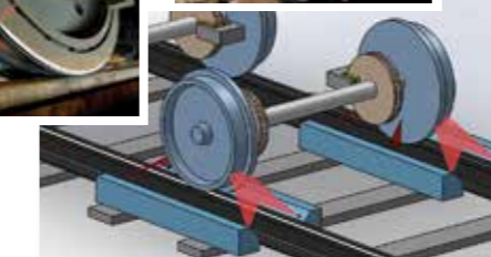
Profil et diamètre / profile & diameter
